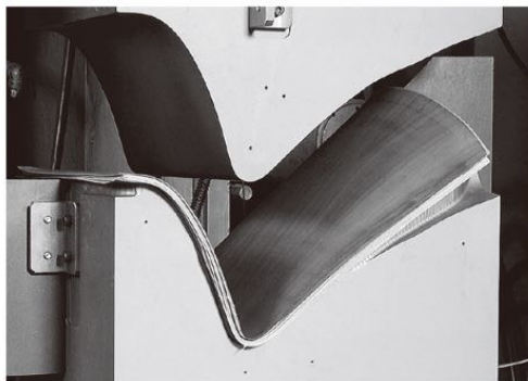
バタフライスツール成形の様子
